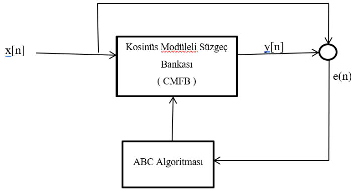
Şekil 3. CMFB tasarım şeması
