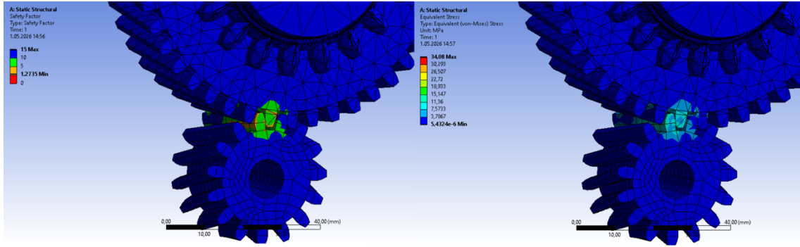
Şekil 10. PLA malzemesi tanımlanmış helis dişli çiftinin güvenlik faktörü ve eşdeğer von-Mises gerilmesi (1000 Nmm moment pinyon dişliye uygulanmakta)
