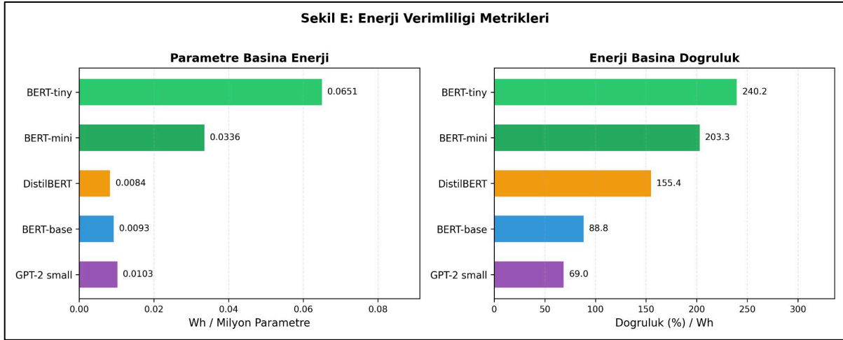
Şekil 5. Enerji Verimliliği Metrikleri (Sol: Parametre başına enerji, Sağ: Enerji başına doğruluk)
