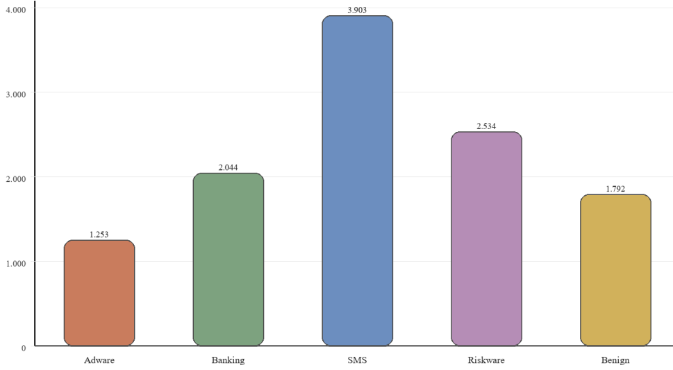
Şekil 2. Temizlenmiş CICMalDroid2020 tabanlı veri kümesinin sınıf dağılımı.
