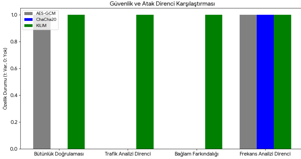
Şekil 2. Siber Saldırı Direnci ve Güvenlik Özellikleri Karşılaştırması
