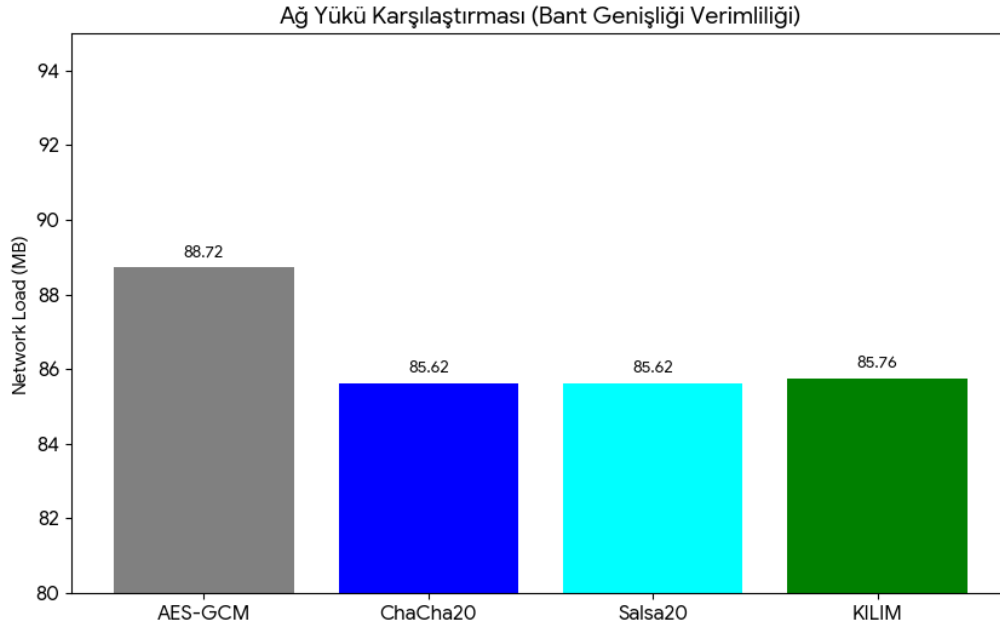
Şekil 1. Algoritmaların Toplam Ağ Yüğü Performansı (MB)
