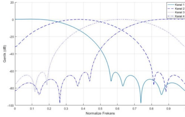
Şekil 4. 4 kanal için CMFB genlik yanıtı
