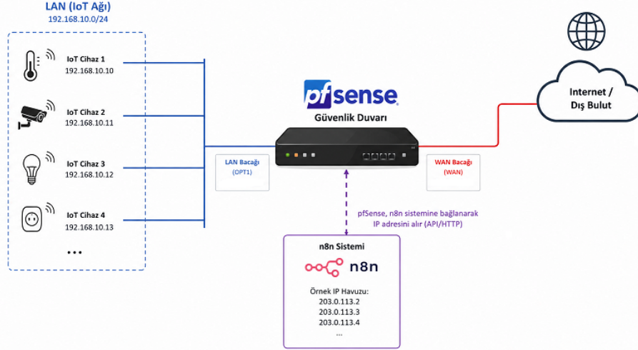
Şekil 1. Tasarlanan ağ diyagramı
