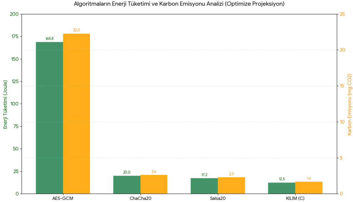
Şekil 3. Yazılımsal Optimizasyonun Enerji ve Karbon Emisyonu Üzerindeki Projeksiyonu
