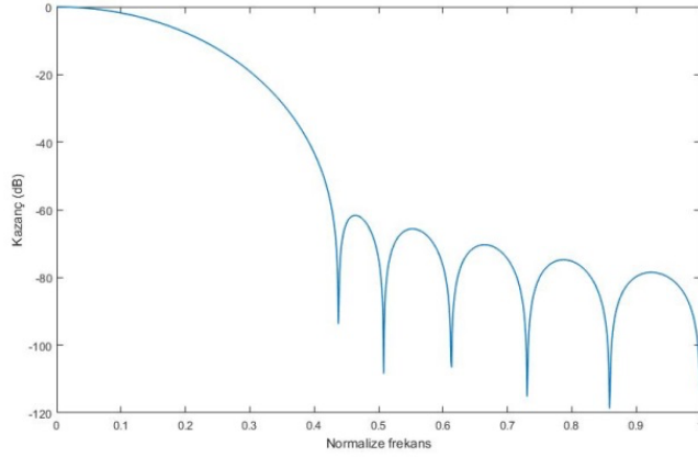
Şekil 4. CMFB prototip süzgeç logaritmik genlik yanıtı
