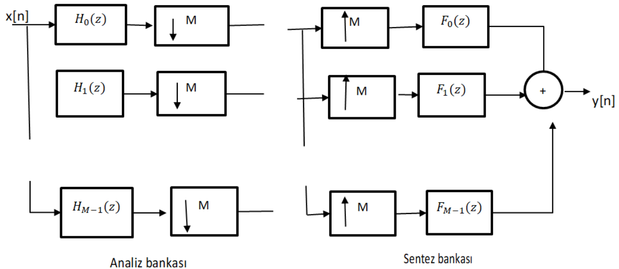
Şekil 1. M kanallı CMFB yapısı
