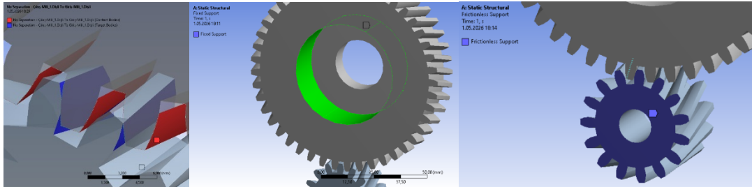
Şekil 4. Sınır şartlarının belirlenmesi kapsamında bağlantılar ve sabitlenen kısımlar
