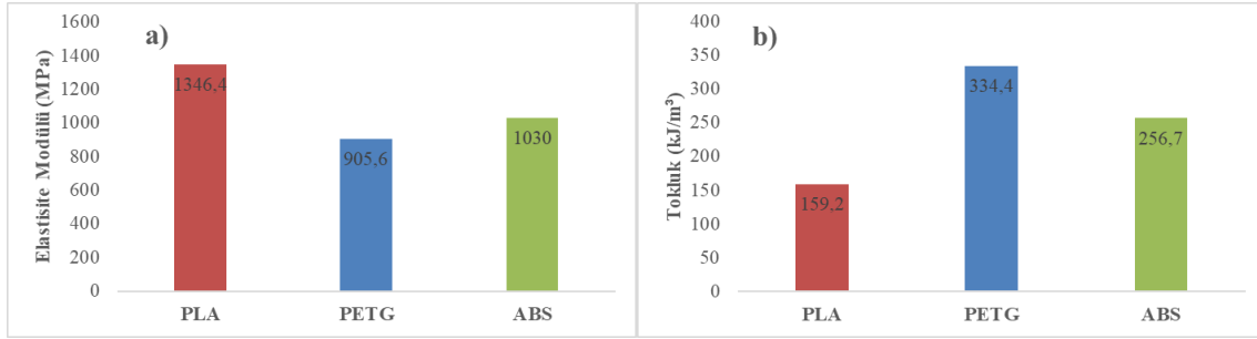
Şekil 9. Test edilen malzemelerin elastisite modülü (a) ve tokluk (b) değerleri
