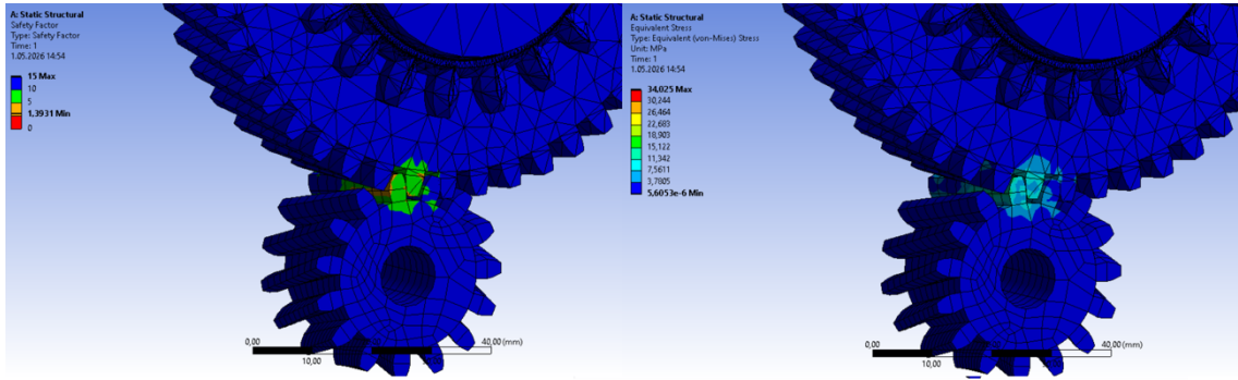
Şekil 11. PETG malzemesi tanımlanmış helis dişli çiftinin güvenlik faktörü ve eşdeğer von-Mises gerilmesi (1000 Nmm moment pinyon dişliye uygulanmakta)
