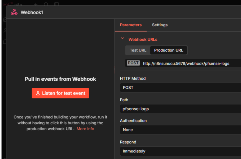
Şekil 3. Pfsense'ten log kaydının alınacağı N8n Webhook düğümü
