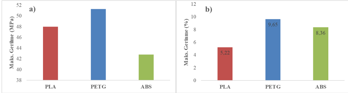
Şekil 8. Test edilen malzemelerin maksimum gerilme (a) ve gerinim (b) değerleri
