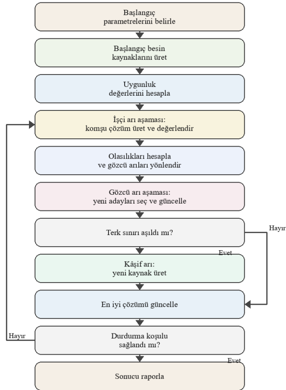
Şekil 1. Yapay Arı Kolonisi algoritmasının temel akışı (Karaboğa, 2010: s.6915 temel alınarak yazar tarafından yeniden çizilmiştir).
