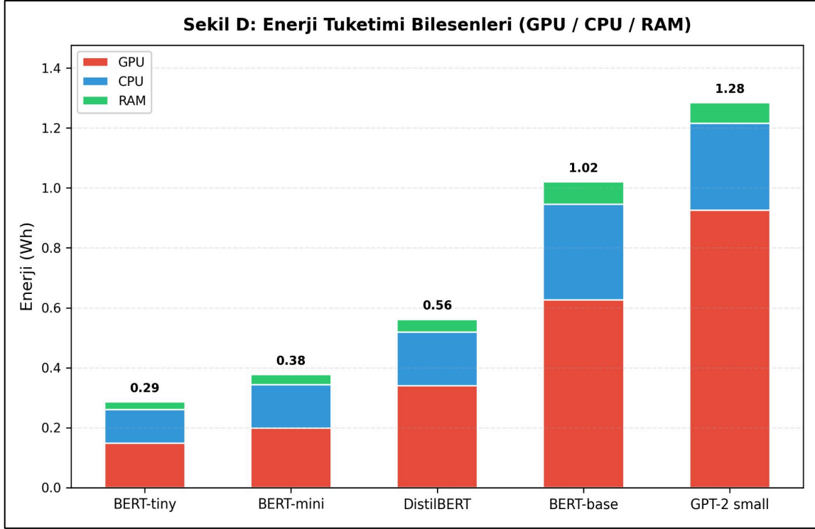
Şekil 3. Enerji Tüketimi Bileşenleri (GPU / CPU / RAM)
