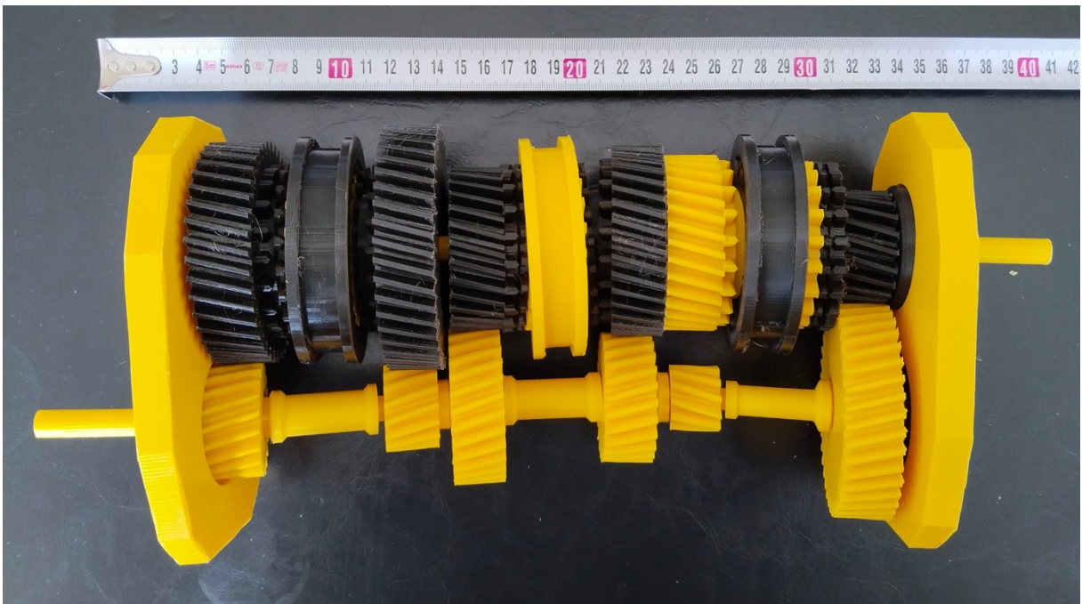
Şekil 7. 3B yazıcı ile üretilen parçaların montajlanmış son hali
