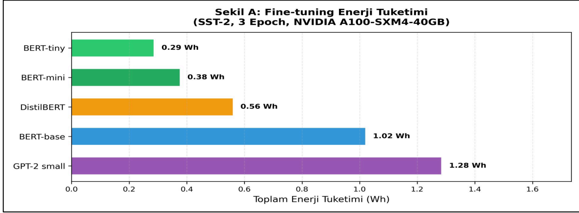
Şekil 1. Fine-tuning Enerji Tüketimi (SST-2, 3 Epoch, NVIDIA A100)
