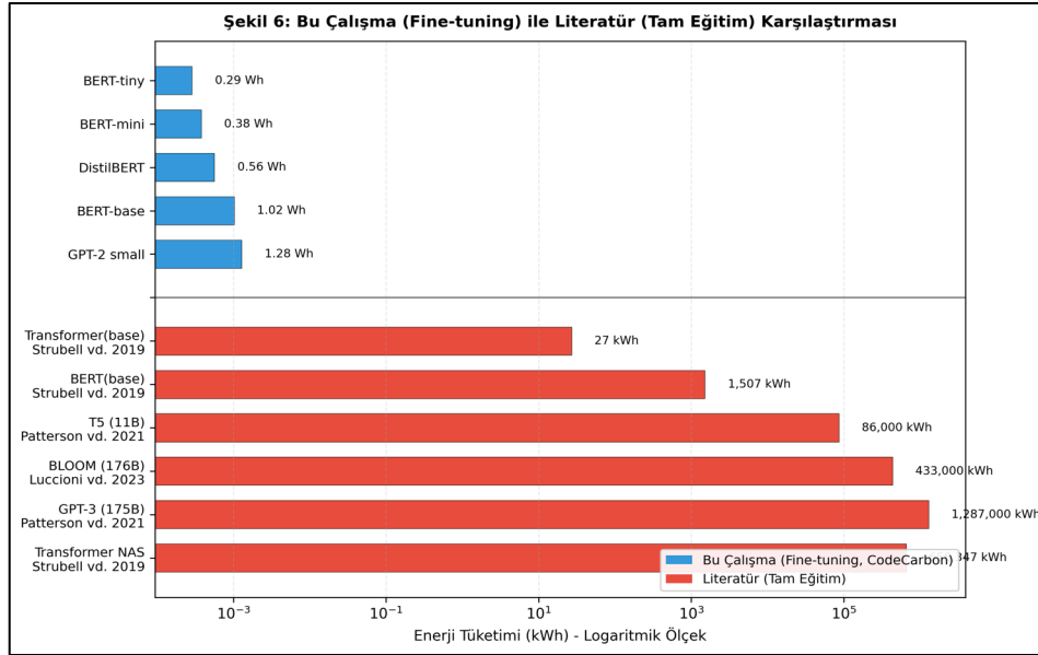
Şekil 6. Bu Çalışma (Fine-tuning) ile Literatür (Tam Eğitim) Enerji Tüketimi Karşılaştırması (Logaritmik Ölçek)
