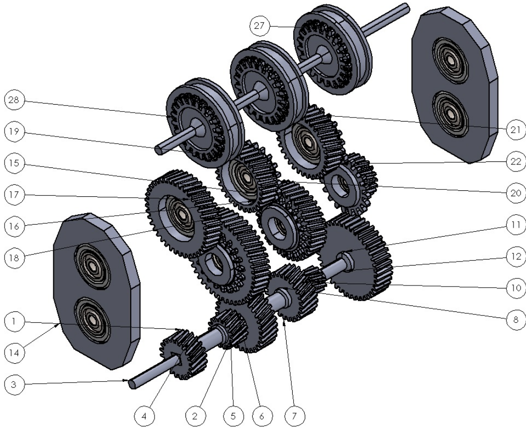
Şekil 2. Montaj resmin patlatılmış görünümü (öge numaralarına karşılık tanımlar Tablo 2.1’de verilmiştir)
