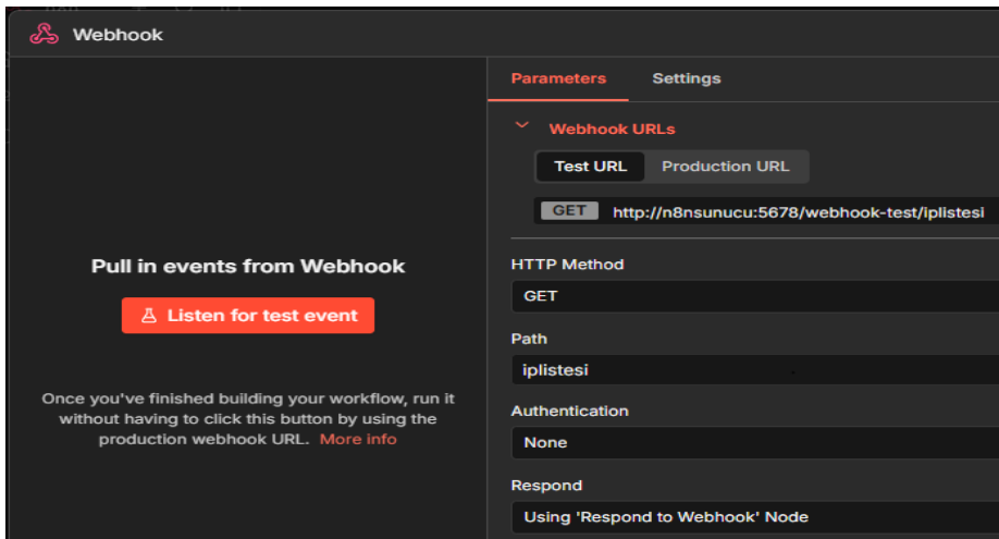
Şekil 5. N8n Webhook IP listesi bağlantısı
