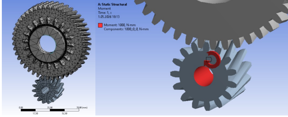
Şekil 5. Analiz öncesi mesh ve moment uygulaması
