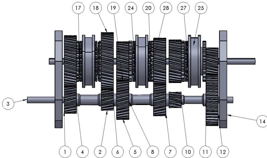
Şekil 1. 5 geçişli şanzımanın montaj resmi (öge numaralarına karşılık tanımlar Tablo 1’de verilmiştir)
