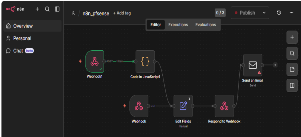
Şekil 4. N8n üzerinde tasarlanan iş akış diyagramı
