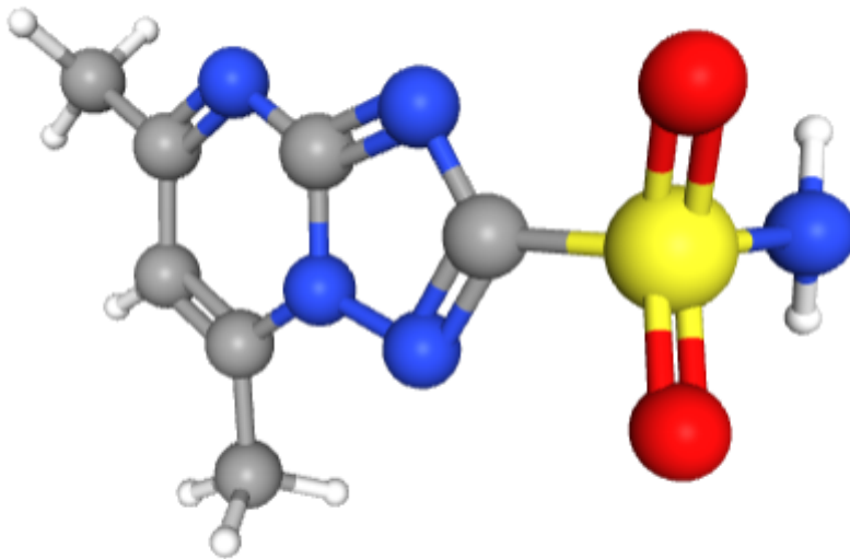
Şekil 1. Molekülün optimize yapısı.
