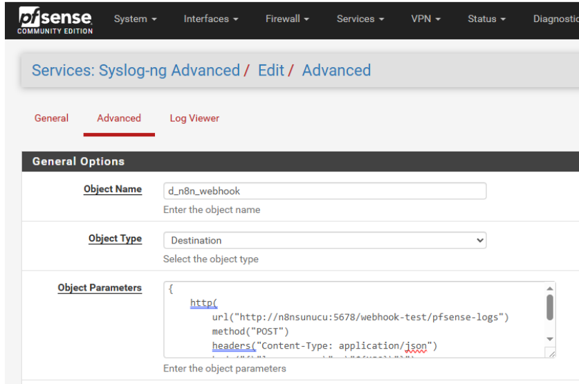
Şekil 2. Pfsense log kaydının N8n sunucusuna gönderimi
